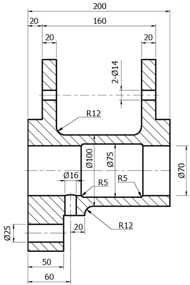
KESİT A-A
