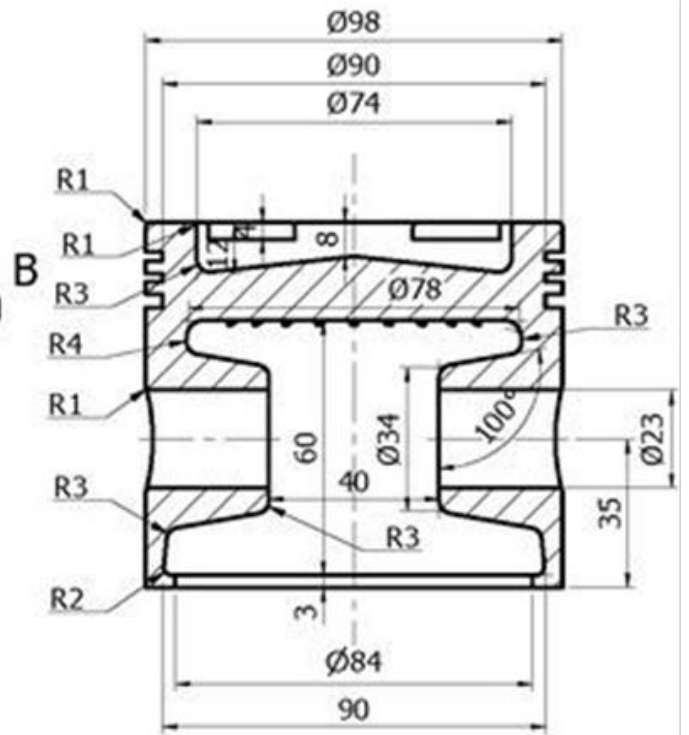
KESİT A-A
