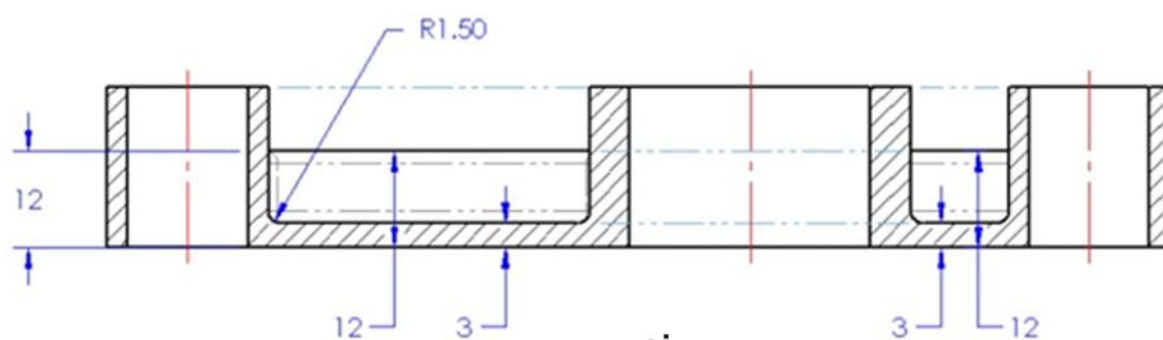
KESİT A-A
